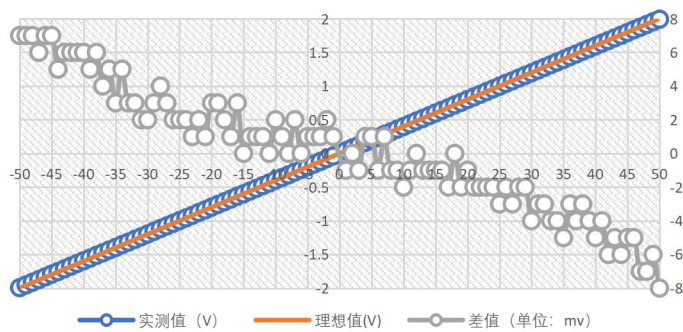
图 8: 线性输出 vs. IP 误差图
