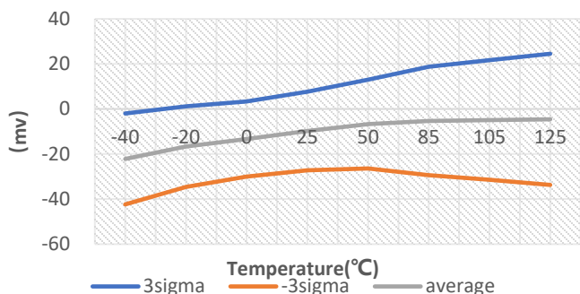
图 3: 零点输出电压温漂
