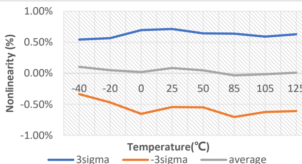
图 6: 非线性误差温漂
