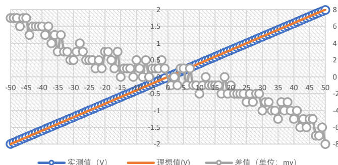
图 8: 线性输出 vs. IP 误差图
