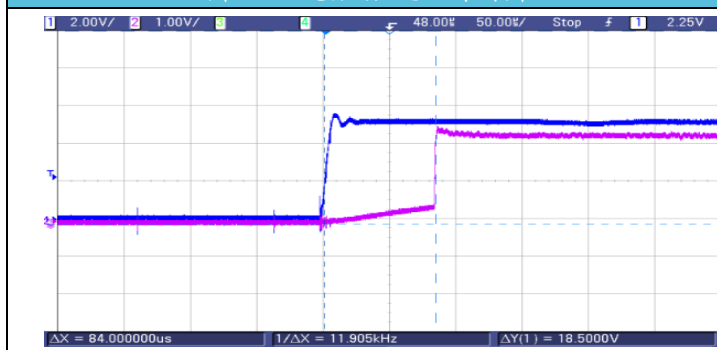
图 7: 上电启动 POR 时间图
